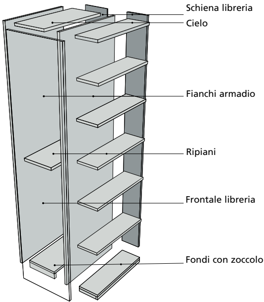
Terminale libreria con anta apribile
