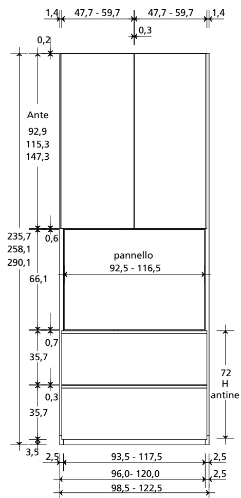
PROSPETTO CON FRONTALI
