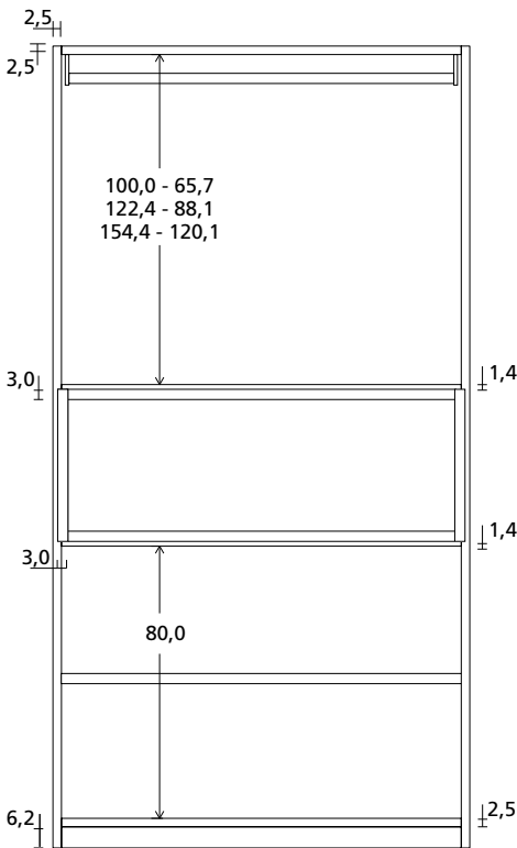
PROSPETTO SENZA FRONTALI
