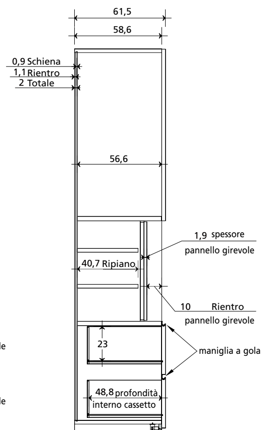
VISTA LATERALE
