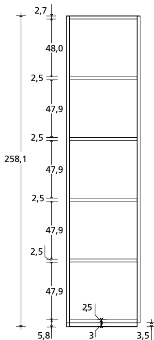
VISTA LATERALE
