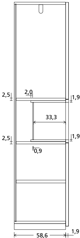
VISTA LATERALE
