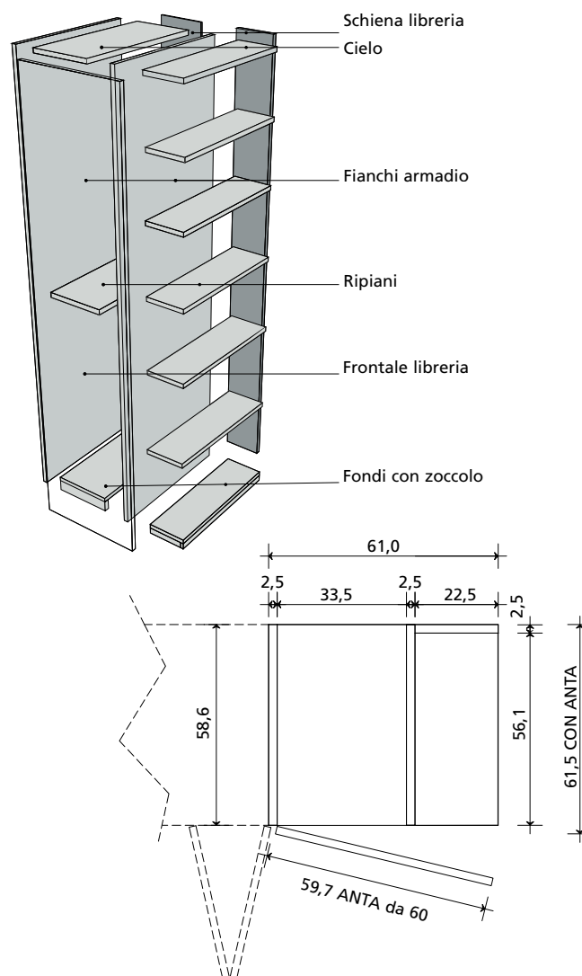
VISTA IN PIANTA
