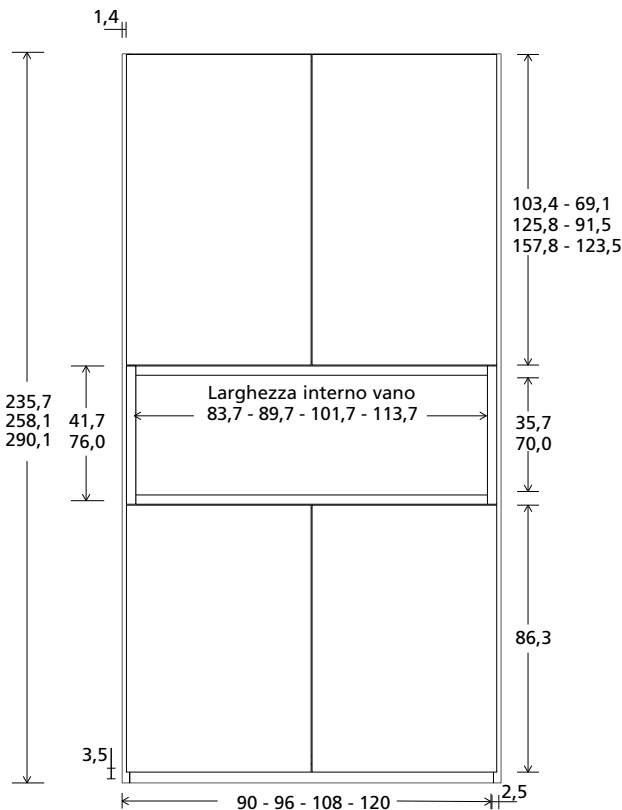
PROSPETTO CON FRONTALI
