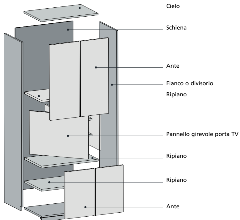
Colonna con 4 antine, e porta TV girevole
