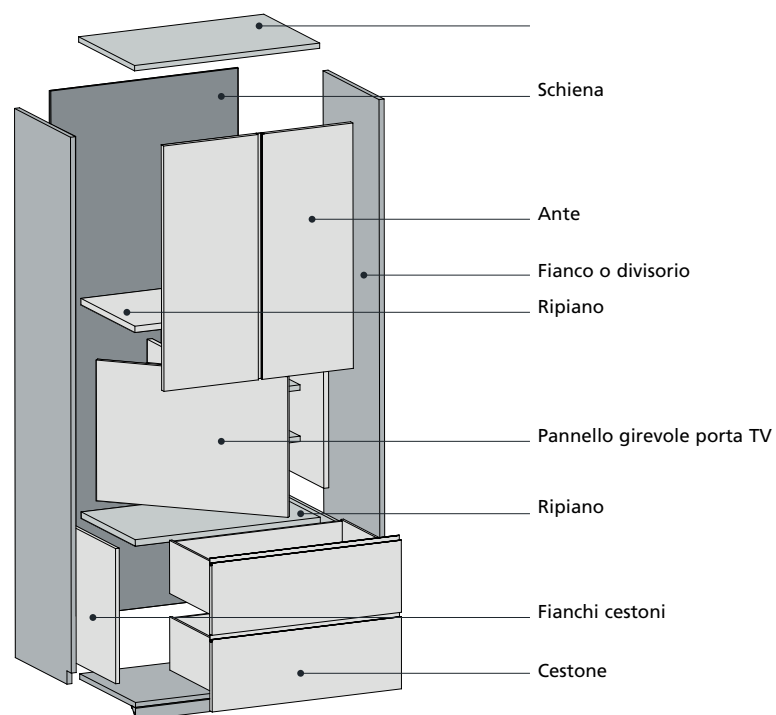
Colonna con 2 cestoni, maniglia a gola con porta TV girevole
